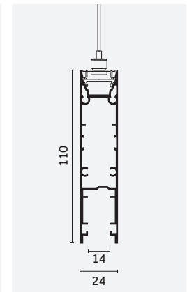
Deep Pendant
