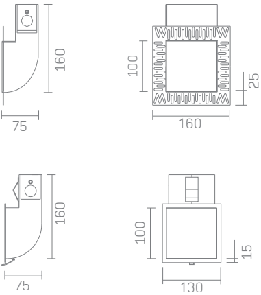
bezel
