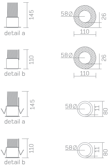
bezel
